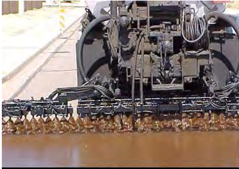
Figure 3–13 : Épandeur d’asphalte procédant à l’application d’une émulsion; vue de l’arrière. L’émulsion est habituellement de couleur brune et devient noire à mesure que se fait la cure de l’émulsion. Les buses de la rampe d’épandage assurent de multiples recouvrements de la surface.
