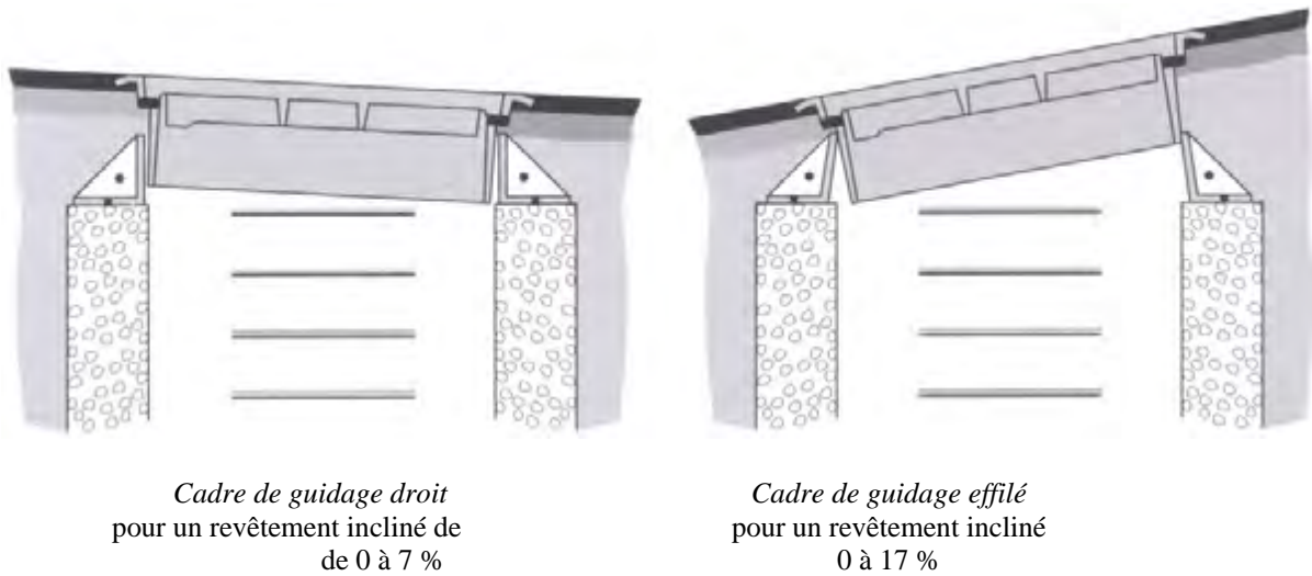
Figure 3-1 : Tampons réglables avec cadre de guidage (droit ou effilé).
