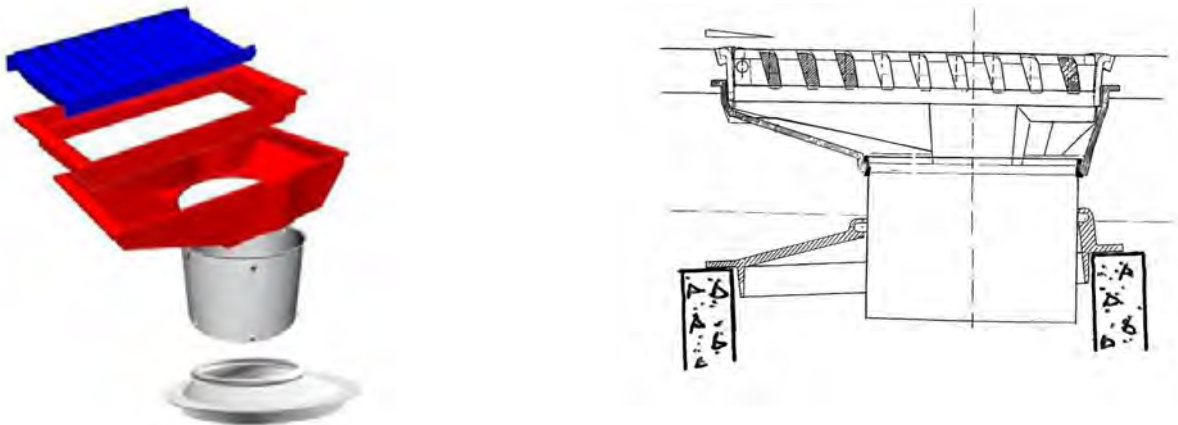
Figure 3-2 : Autre type de cadre et de tampon réglables.
